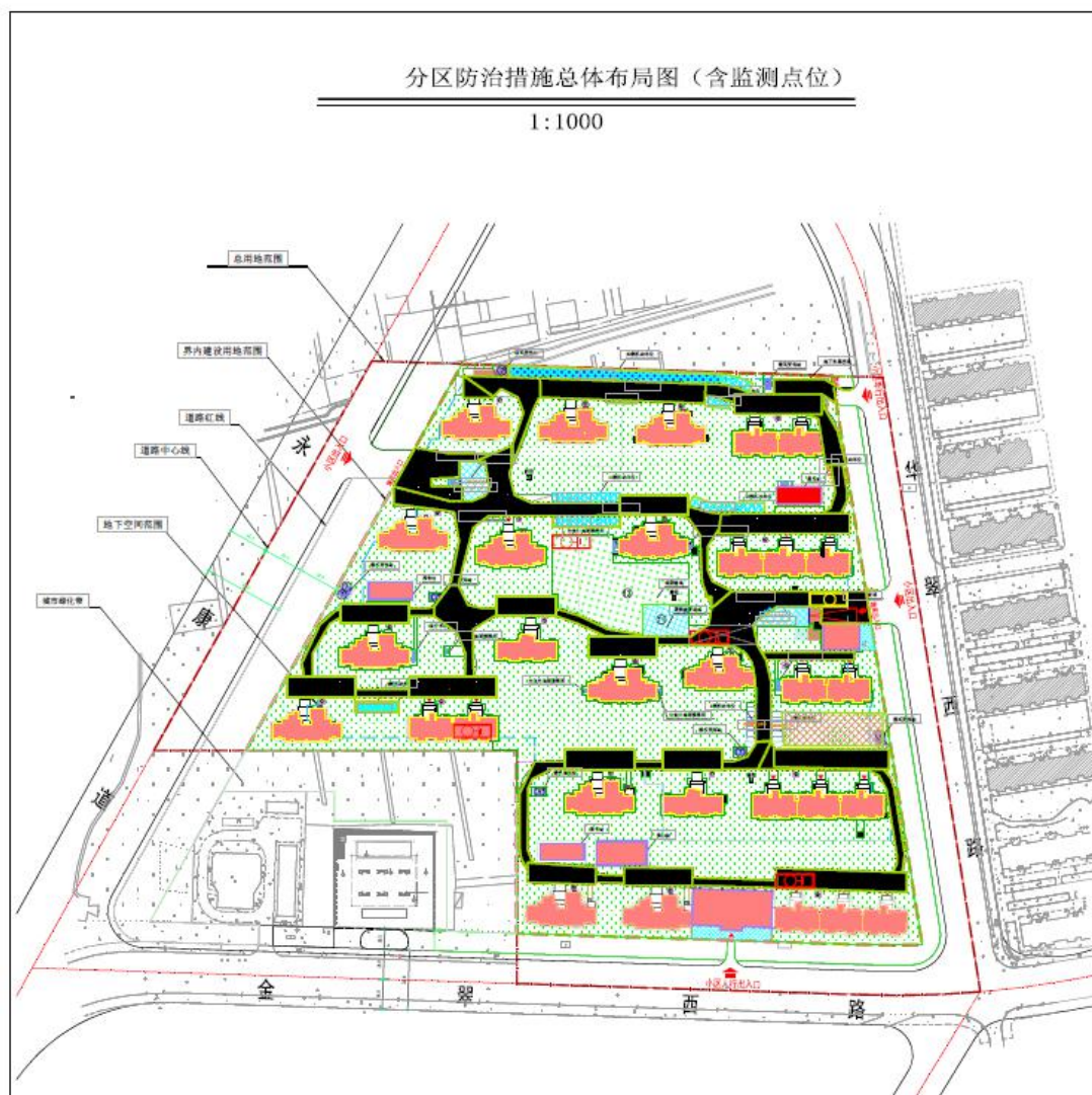
附图 2. 监测分区及监测点布设图
